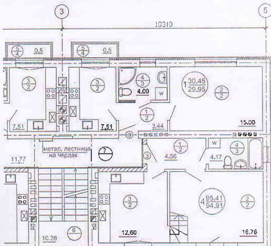
План отделочных работ 5 этажа.
